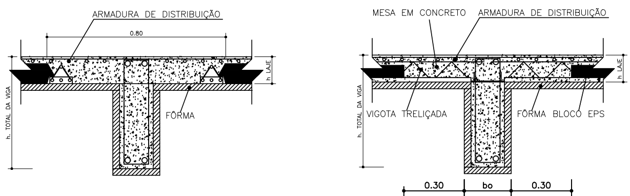
DETALHE 04 DETALHE ENCHIMENTO DAS VIGAS "T", "L" SEM ESCALA
