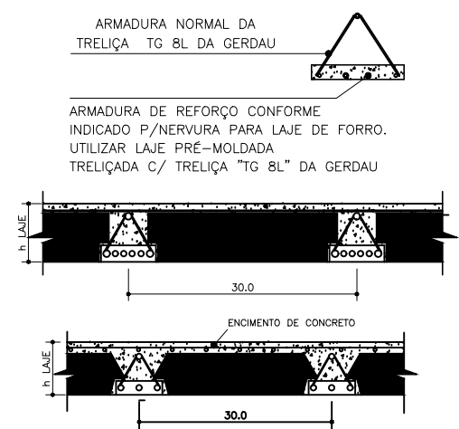
DETALHE 02 REFORÇO DA TRELIÇA DA LAJE SEM ESCALA
