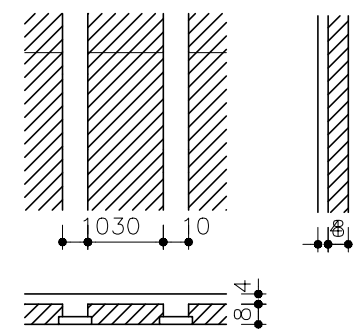
DETALHE 01 CORTE DAS LAJES SEM ESCALA
