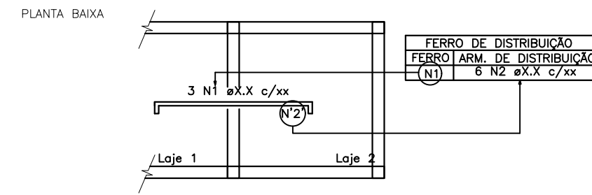
DETALHE 05 ARMADURA DE CONTINUIDADE DA LAJE E MONT. DA ARM. DE DISTRIBUIÇÃO SEM ESCALA
