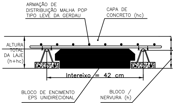
DETALHE 03 DETALHE VIGOTA SIMPLES SEM ESCALA
